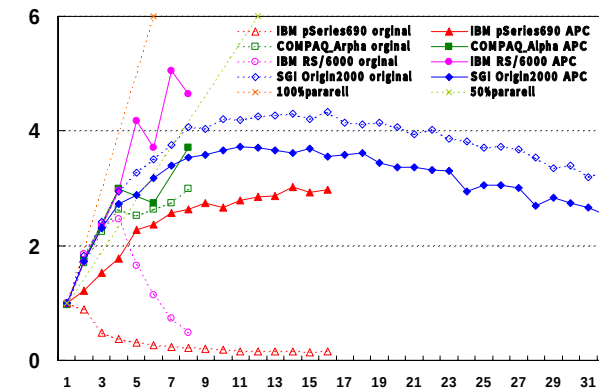
103.su2cor (Hierarchical)
